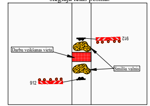
Būvdarbu vietas lokālais aprikojums caurbraukšanai slēgtajā ielas posmā.
