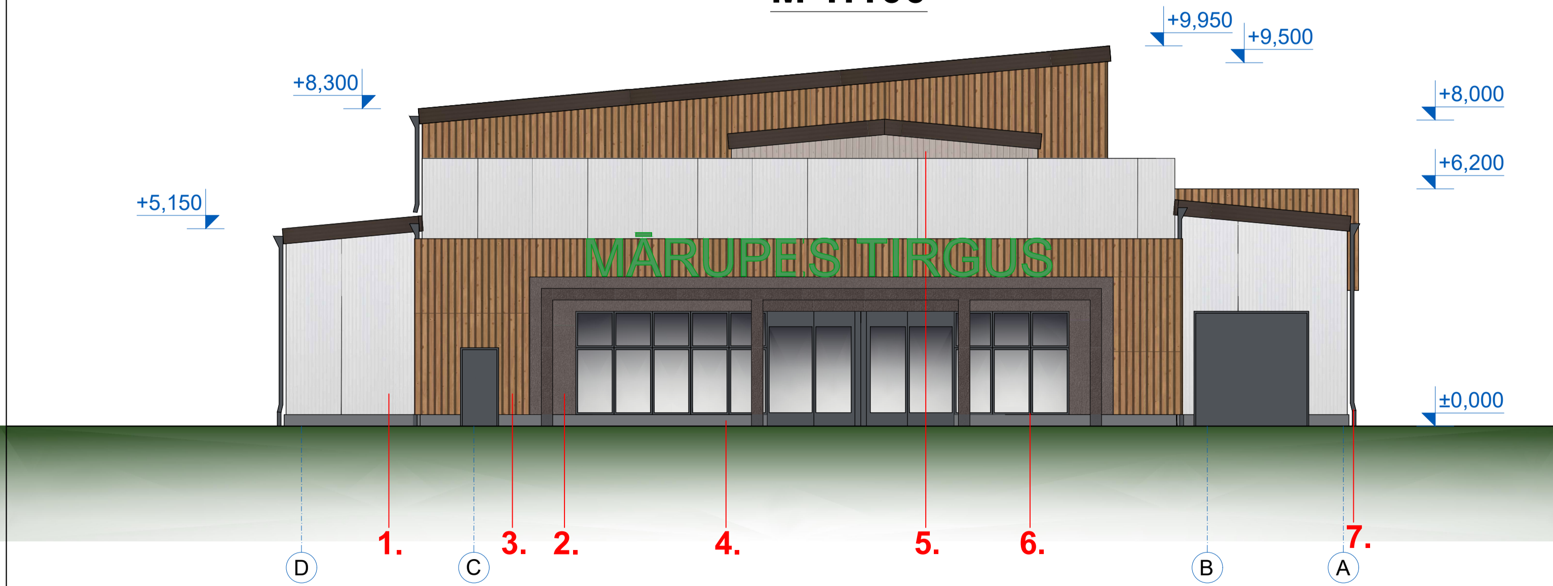
FASĀDE ASĪS D-A M 1:100
