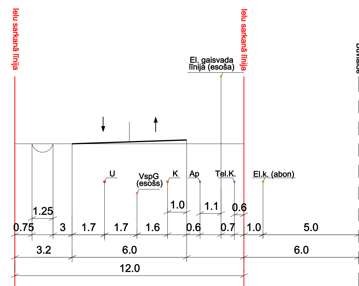
M 1:400 Ielas griezumums A-A
