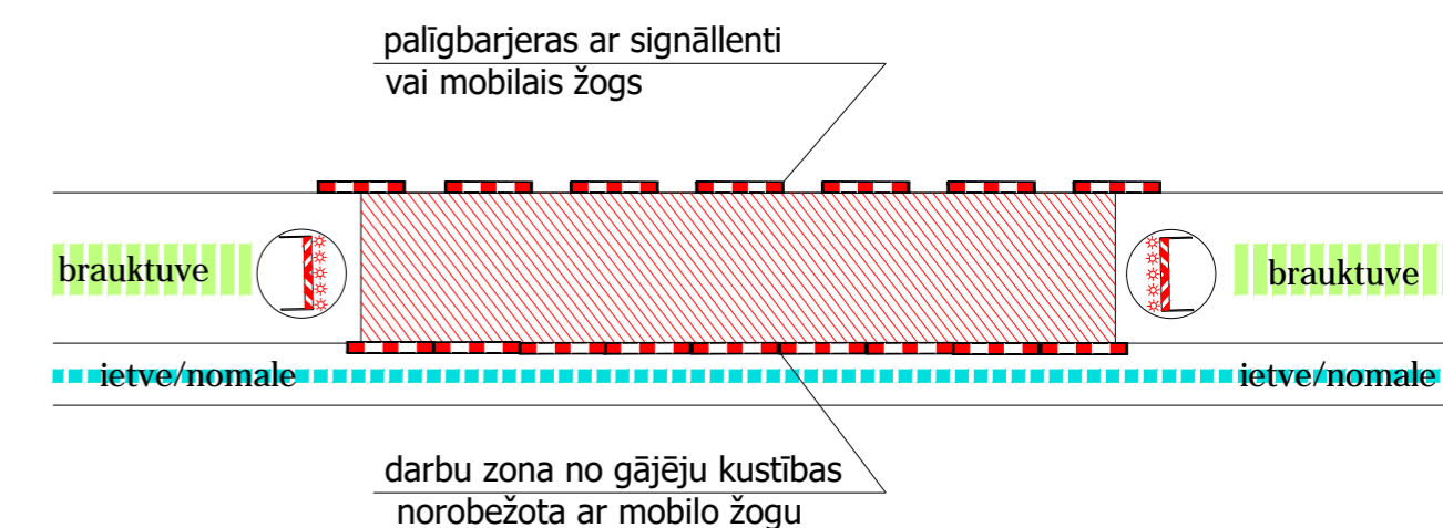
Shēma Nr.1
