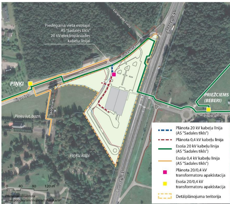
22.attēls. Principiālais elektroapgādes risinājums
