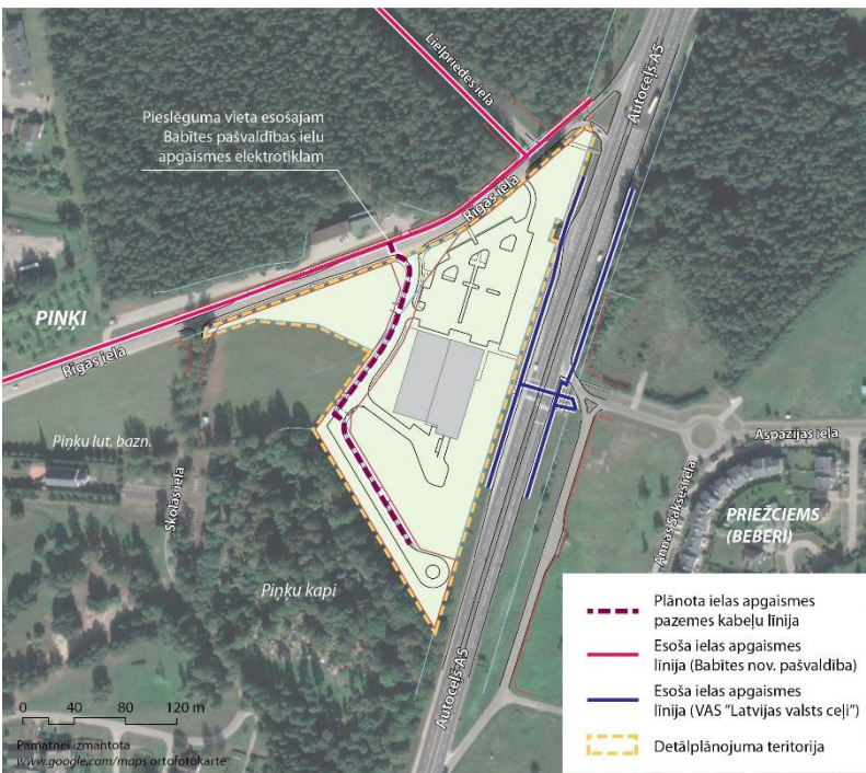
23.attēls. Principiālais apgaismes risinājums
