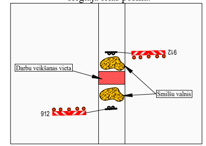
Būvdarbu vietas lokālais aprīkojums caurbraukšanai slēgtajā ielas posmā.
