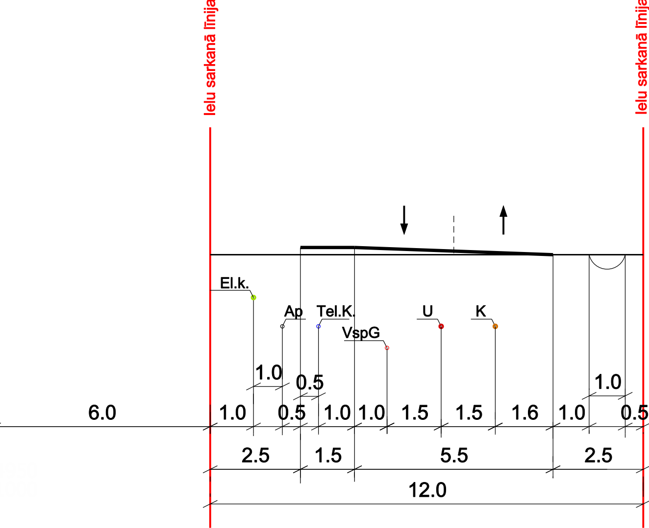
Ielas griezumums A-A M 1:400
