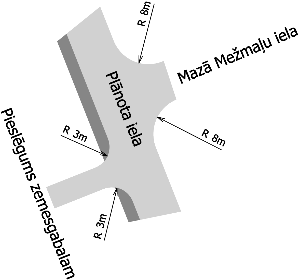
Ielu pieslēgumu noapaļojumu rādus
