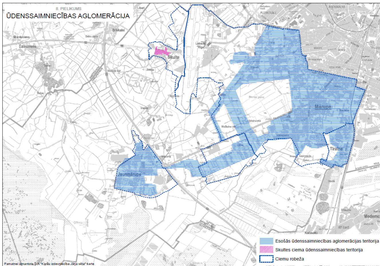
30. attēls. Ūdenssaimniecības aglomerācijas tīkls. Mārupes novada teritorijas plānojuma 2014.-2026.gadam grozījumu redakcija (projekts, 2019).
