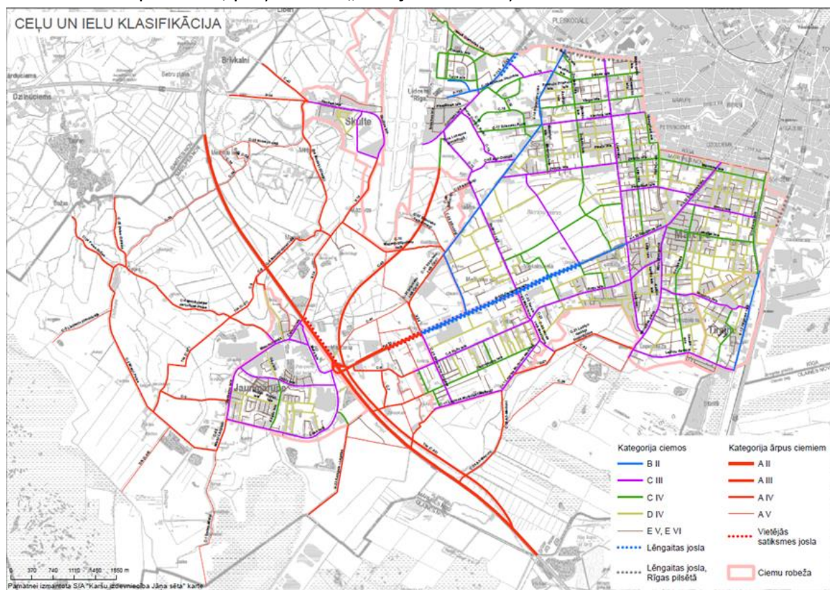
24. attēls. Ielu un ceļu klasifikācija. Mārupes novada teritorijas plānojuma 2014. - 2026. gadam grozījumu redakcija (projekts, 2019)
