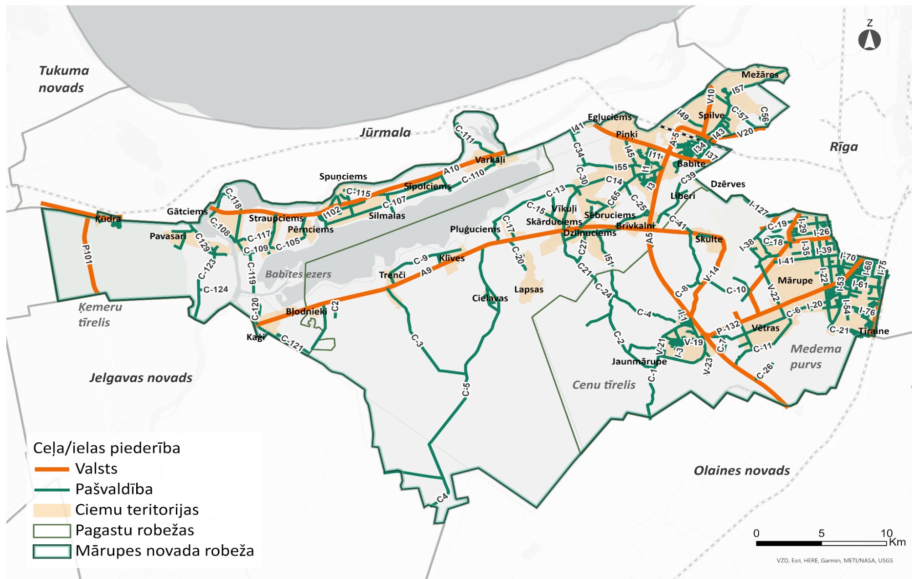
Attēls Nr.19 Valsts un pašvaldības ceļu tīkls Mārupes novadā
