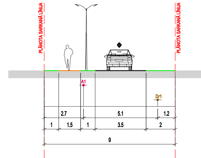
PERSPEKTĪVĀ IZBŪVĒJAMĀ IELAS POSMA ŠĶĒRSPROFILS GRIEZUMS 2 - 2
