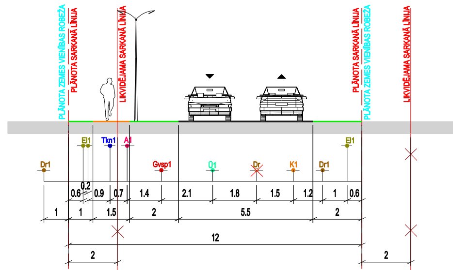
PLĀNOTĀS IELAS ŠĶĒRSPROFILS GRIEZUMS 1 - 1
