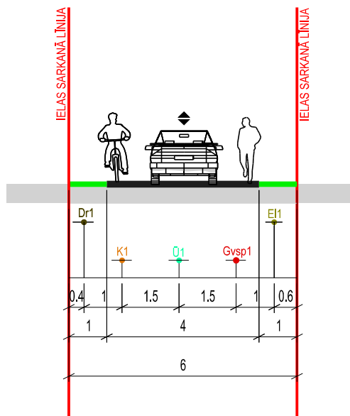
E V KATEGORIJAS 6 METRUS PLATO IELU TEORĒTISKAIS GRIEZUMS
