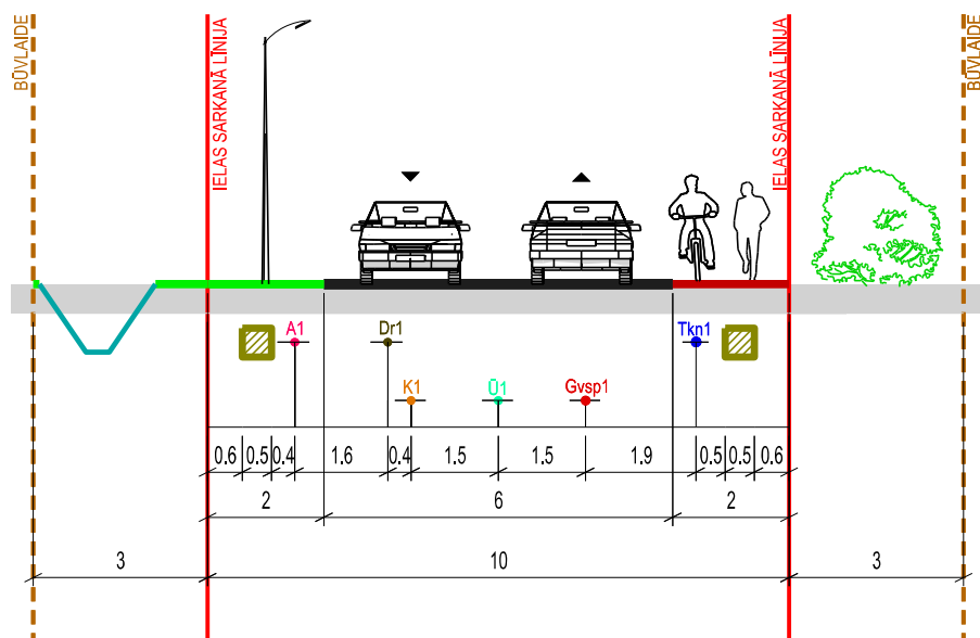
E V KATEGORIJAS 10 METRUS PLATO IELU TEORĒTISKAIS GRIEZUMS
