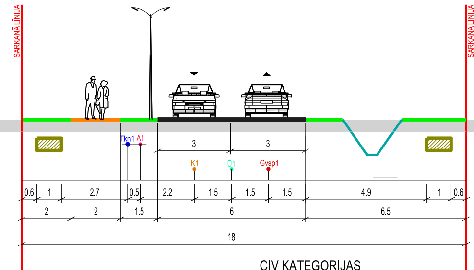
CIV KATEGORIJAS 18 METRUS PLATO IELU TEORĒTISKAIS GRIEZUMS
