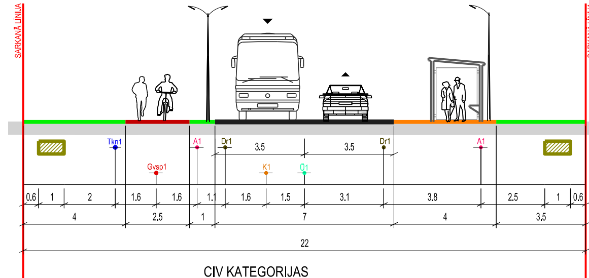
CIV KATEGORIJAS 22 METRUS PLATO IELU TEORĒTISKAIS GRIEZUMS
