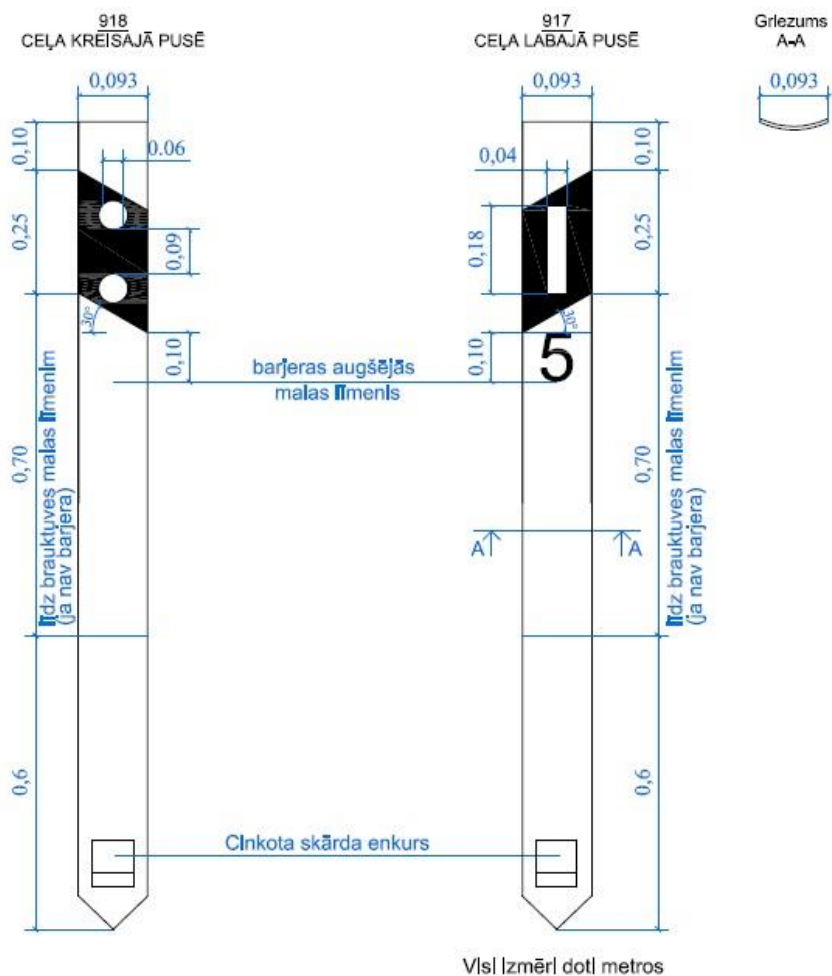
7.4-1 attēls. Signālstabiņi
