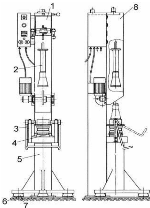
12.8-1 attēls. Triecienu blīvētāja shematiskais attēls
