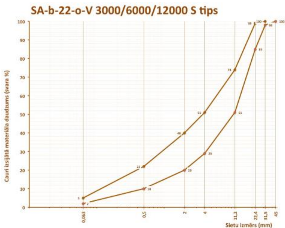
6.3-25 tabula. Prasības mīkstā asfalta SA-b-22-o-V 3000/6000/12000 S tips maisījuma granulometriskajam sastāvam
