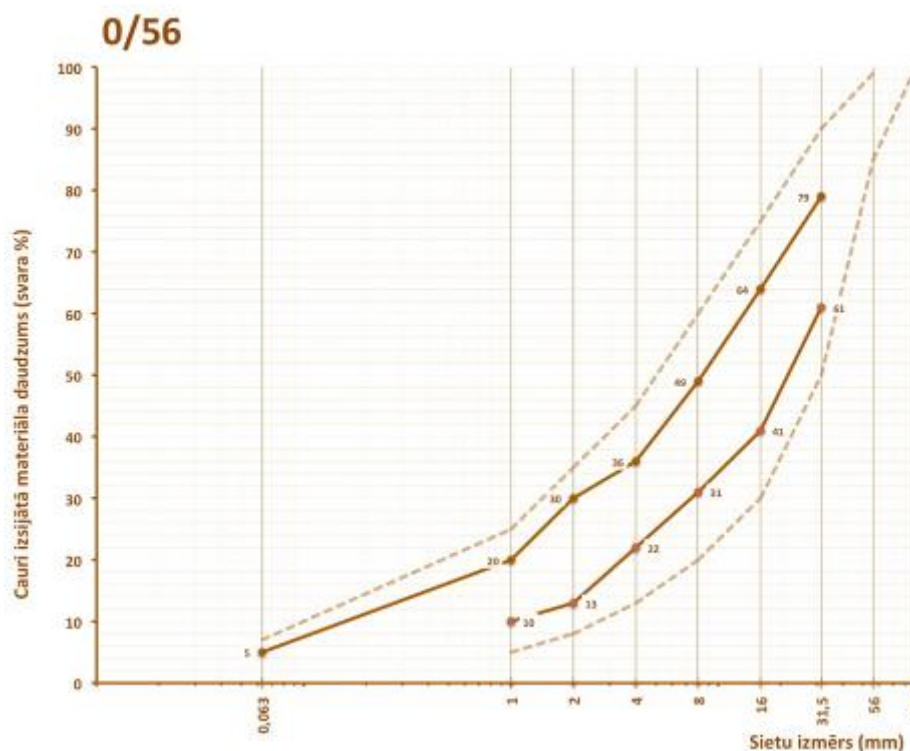
5.2-19 tabula. Prasības 0/56 maisījuma granulometriskajam sastāvam Kopīgā granulometriskā sastāva diapazona kategorija – G C
